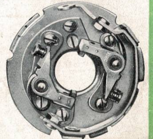
Ruttore "KING DUPLEX"
